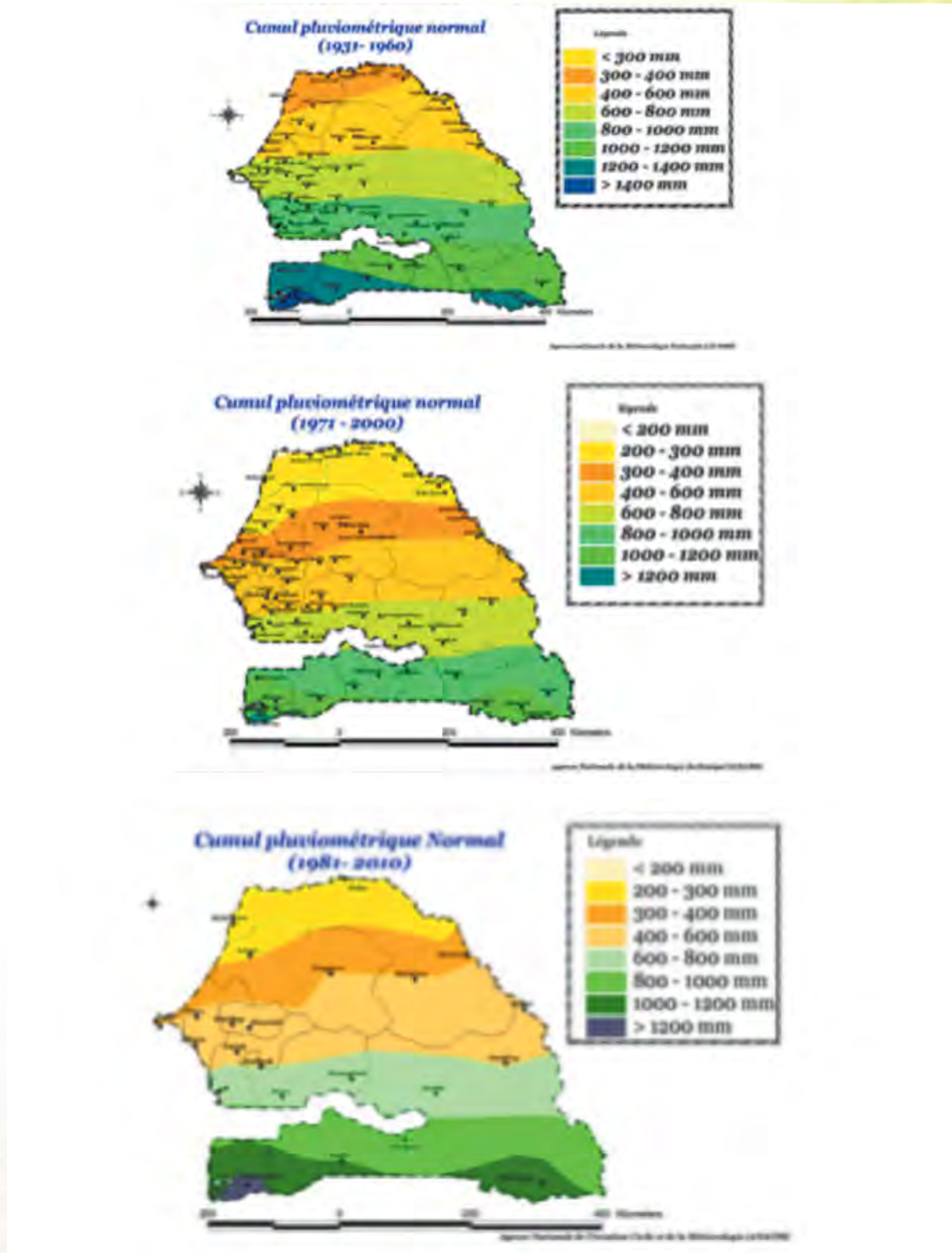
Figure 2 : Normales pluviométriques de 1931-1960, 1971-2000 et 1981-2010
