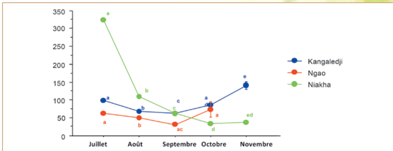
Figure 11 : Evolution de la conductivité électrique de l'eau des mares de Niakha, Kangaledji et Ngao en 2008
