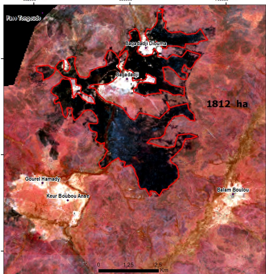
Figure 1 : Cas de feu observés par satellite sur le Sénégal du 10 au 16 avril 2023
