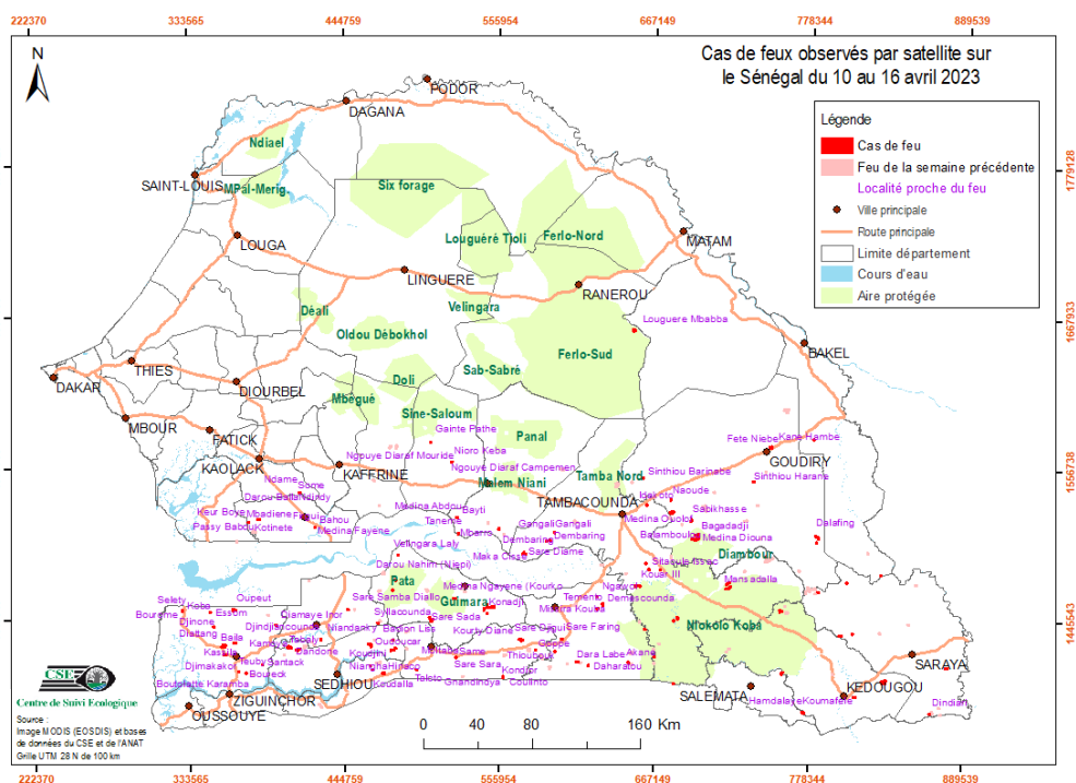
Figure 1 : Cas de feu observés par satellite sur le Sénégal du 10 au 16 avril 2023
