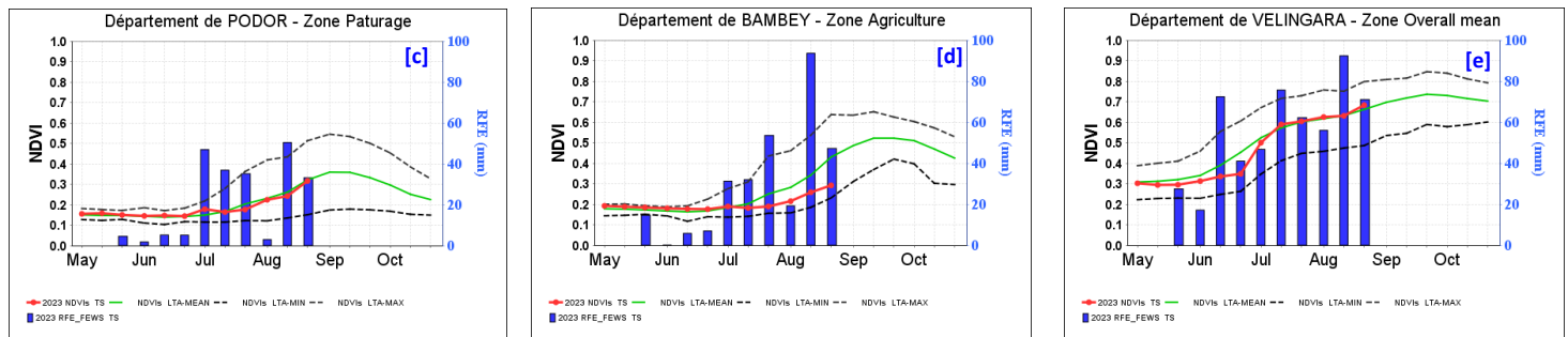
Figure 3 : Evolution du profil du NDVI dans les départements de (c) Podor (zone pastorale), (d) Bambey (zone agricole) et (e) Vélingara (zones pastorale et agricole).
