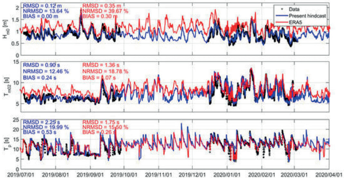
Figure 1 : Validation de nouvelles données rétrospectives de vagues simulées (sur littoral du Sénégal disponible sur les 4 dernières décennies (1980-2021)) à partir de WW3 (en bleu), grâce aux observations de la Bouée MELAX amarrée durant le LMI ECLAIRS-I. Une comparaison est faite avec les Réanalyses de ERA-5 (en rouge) qui sont de moins bonnes résolutions sur la Petite Côte liée à la non prise en compte de la morphologie de la presqu'île de Dakar par ERA-5. (in, Samou et al., 2023a)
