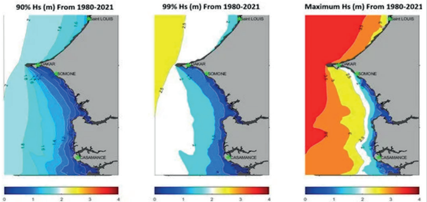
Figure 2 : Ordre de grandeur des Hauteurs significatives (Hs) de vagues pour les 90 ème , 99 ème et 100 ème percentiles des valeurs maximales de vagues en conditions extrêmes sur le littoral sénégalais de 1980 à 2021. (in, Samou et al., 2023a)
